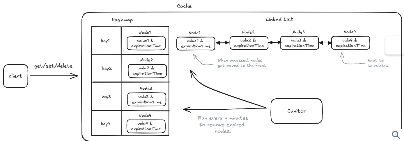
Simple LRU Cache
